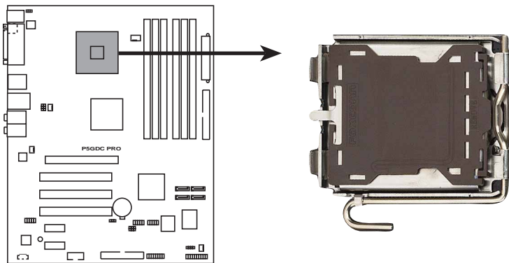
P5GDC PRO CPU Socket 775
