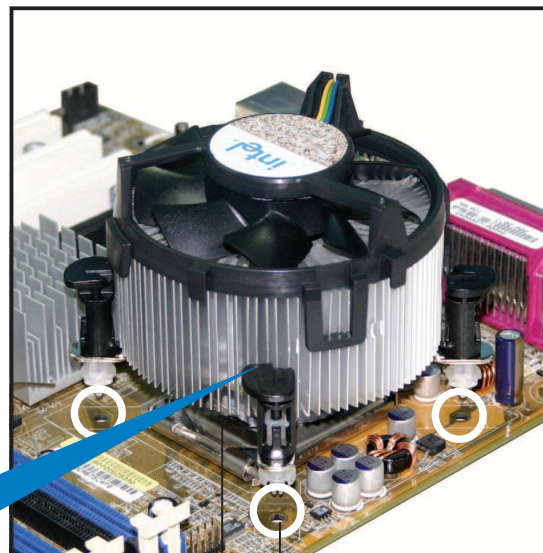
マザーボードの穴 留め具
